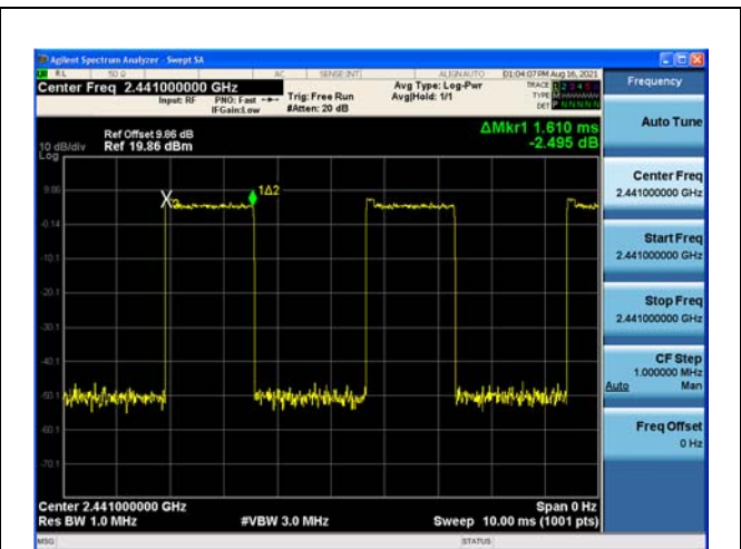
Modulation: \pi/4 DQPSK 2DH3 2441
