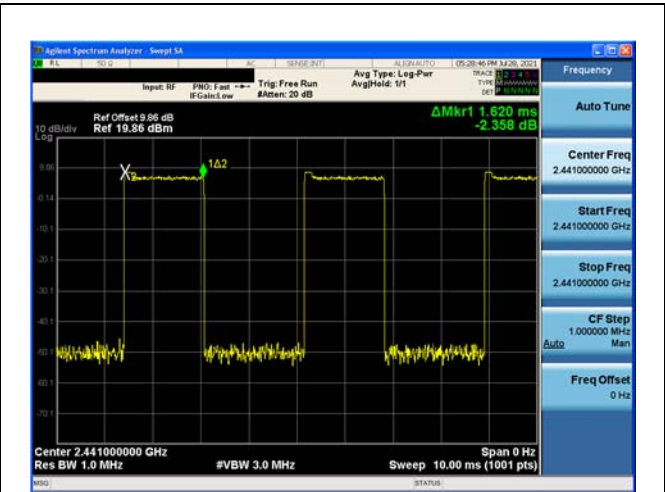
Modulation: \pi/4 DQPSK 2DH3 2441
