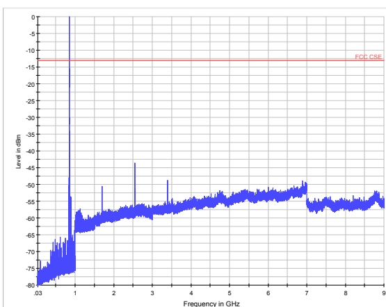
GSM 850 CH-High 30MHz ~ 9GHz
