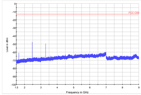
LTE Band 5 10MHz CH-Middle 1.5GHz~9GHz
