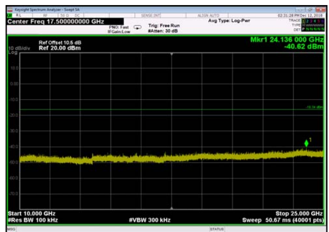
,Plot 5,10000MHz~25000MHz-802.11n(HT40),2452MHz
