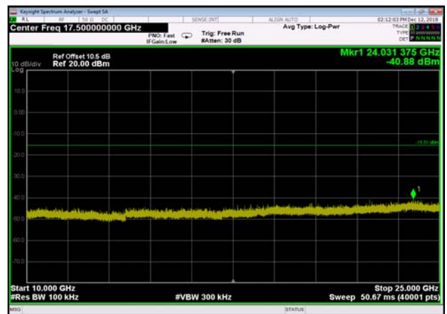
,Plot 5,10000MHz~25000MHz-802.11n(HT40),2452MHz
