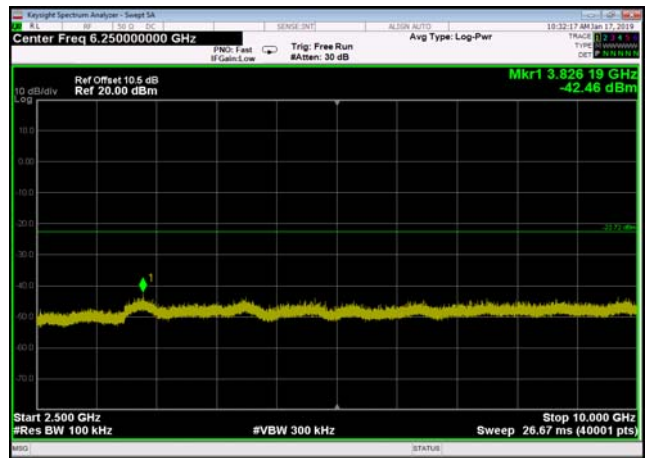
,Plot 4,2500MHz~10000MHz-802.11n(HT20) ,2462MHz,Ant0
