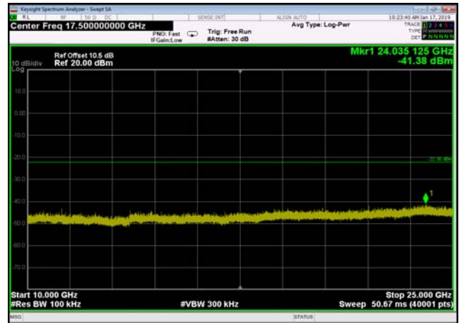
,Plot 5,10000MHz~25000MHz-802.11n(HT2 0),2437MHz,Ant0
