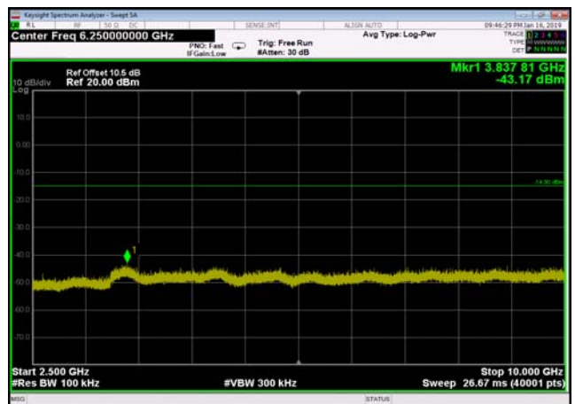
,Plot 4,2500MHz~10000MHz-802.11b ,2462MHz,Ant0
