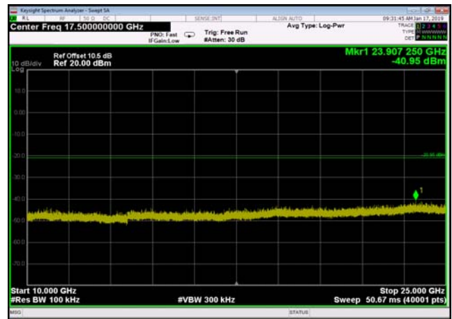
,Plot 5,10000MHz~25000MHz-802.11g ,2462MHz,Ant0
