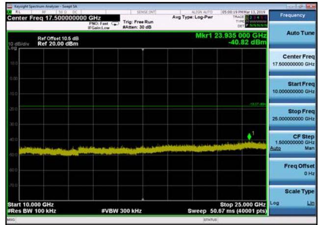
,Plot 5,10000MHz~25000MHz-802.11n(HT2 0),2437MHz
