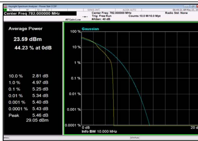
FDD13_10MHz_782MHz_OneRB_high_Q16
