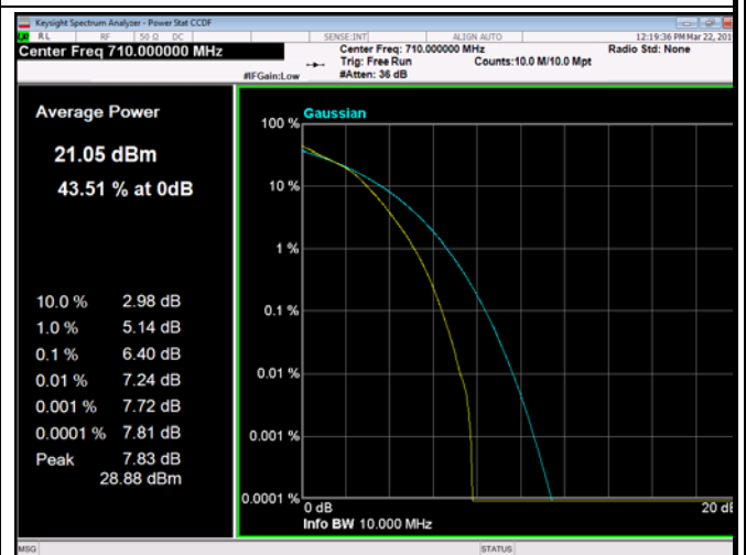
FDD17_10MHz_710_fullRB_Q16
