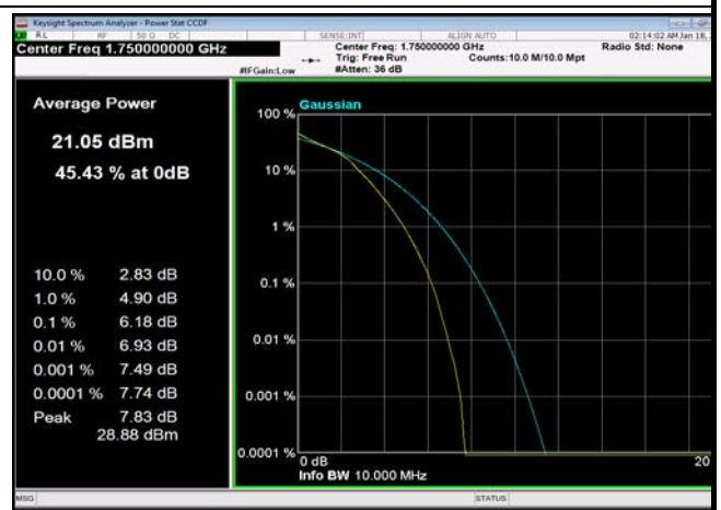
FDD04_10MHz_1750_fullRB_Q16
