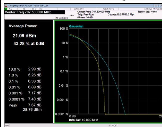
FDD12_10MHz_707.5_OneRB_high_Q16
