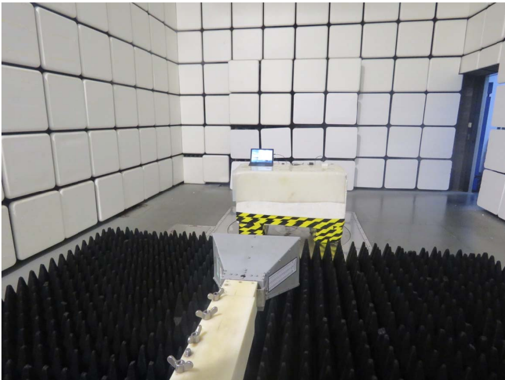
1GHz-18GHz
