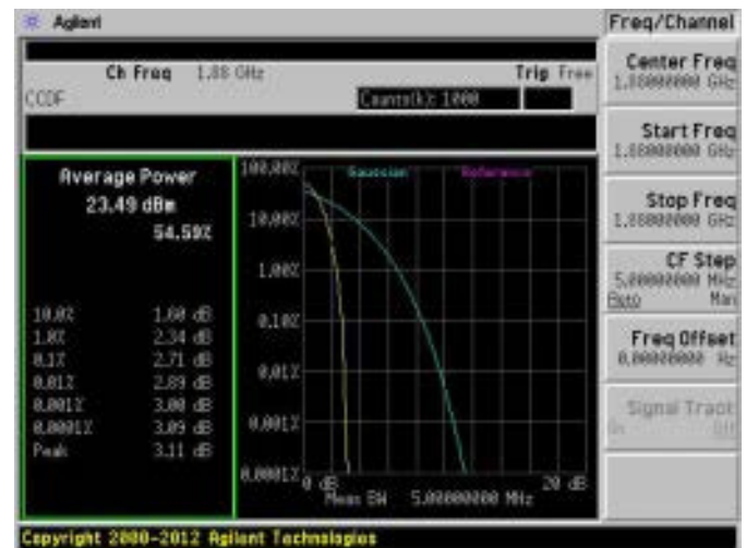
WCDMA Band 2 MCH
