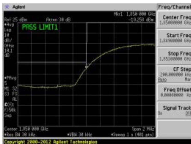
WCDMA Band 2 LCH
