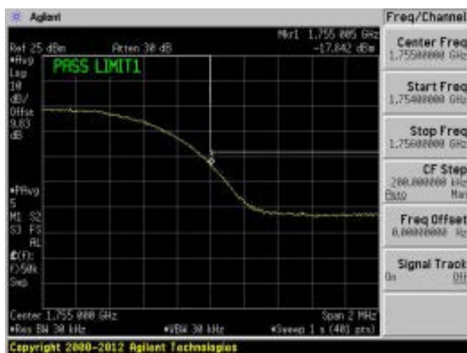
WCDMA Band 4 HCH
