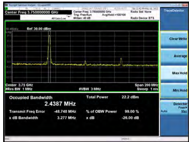
DC_2A-n77(subset 2)A QPSK 1RB 100MHz CH-Middle
