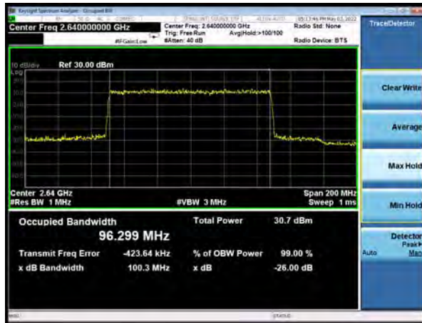
DC_28 A (subset 2)-n41A 16QAM 100%RB 100MHz CH-High
