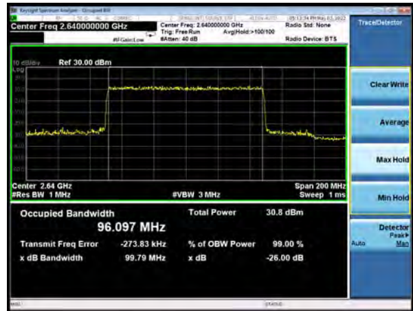
DC_28 A (subset 2)-n41A 64QAM 100%RB 100MHz CH-High
