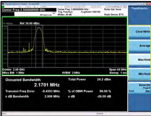
NR n7 16QAM 1RB 20MHz CH-High
