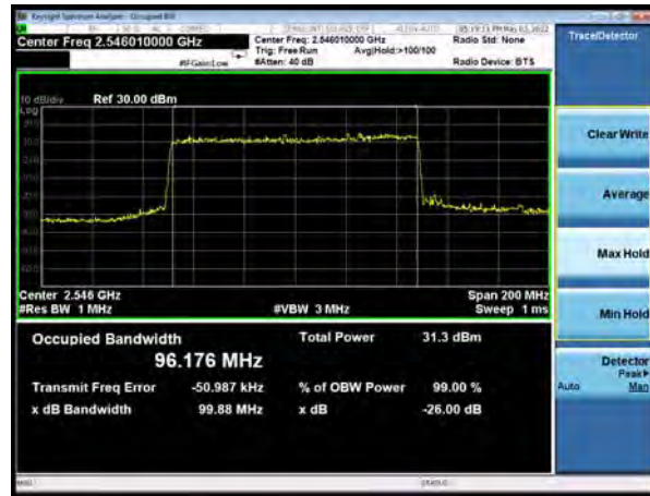
DC_28 A (subset 2)-n41A QPSK 100%RB 100MHz CH-Middle
