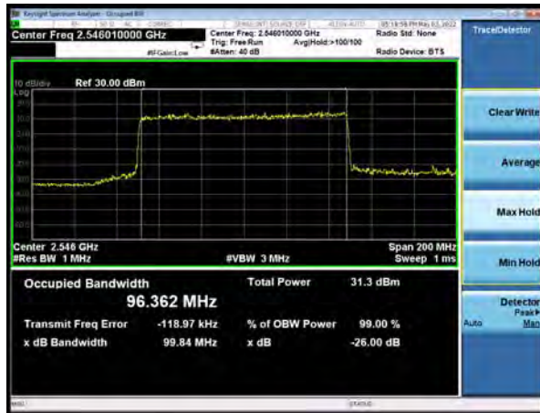
DC_28 A (subset 2)-n41A 16QAM 100%RB 100MHz CH-Middle
