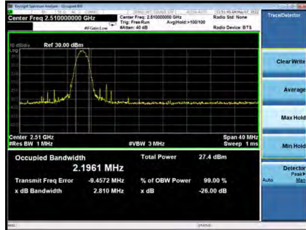
NR n7 64QAM 1RB 20MHz CH-Middle
