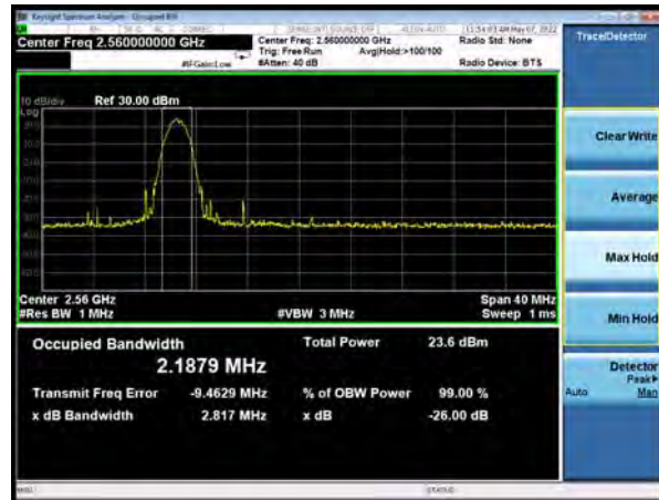
NR n7 64QAM 1RB 20MHz CH-High
