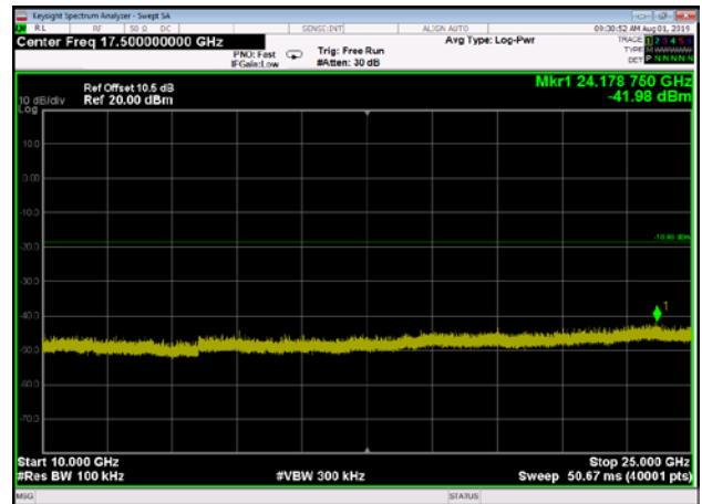
,Plot 5,10000MHz~25000MHz-802.11n(HT40),2452MHz
