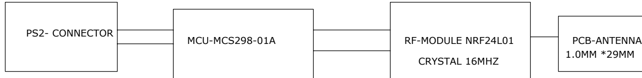
RX-BLOCK DIAGRAM
