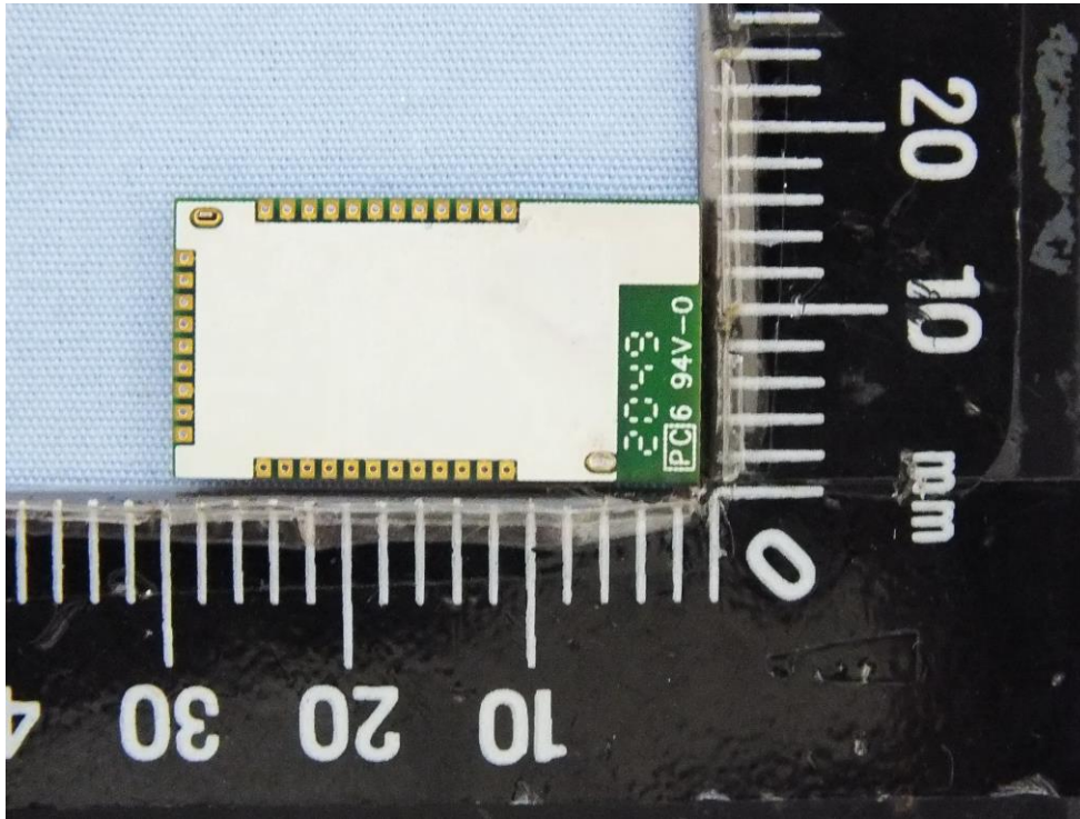
Model: BT740-SA
