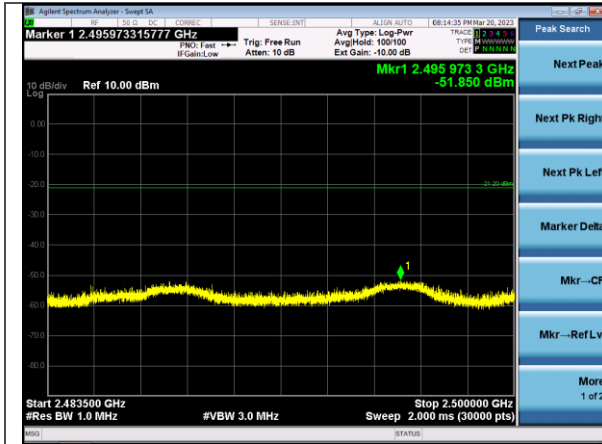
2.4835-2.5 GHz Mid
