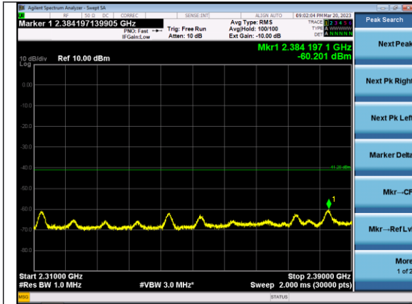
2.31-2.39 GHz Mid
