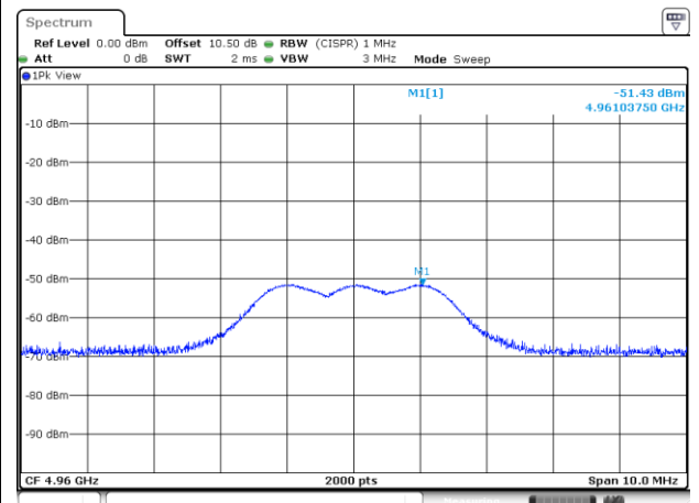
4960MHz - PK
