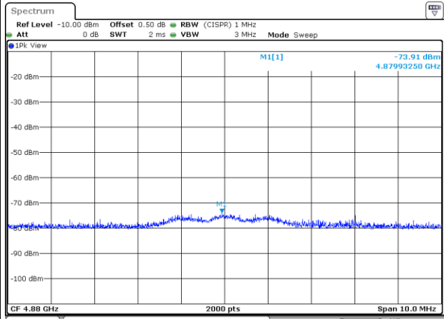
4880MHz - PK
