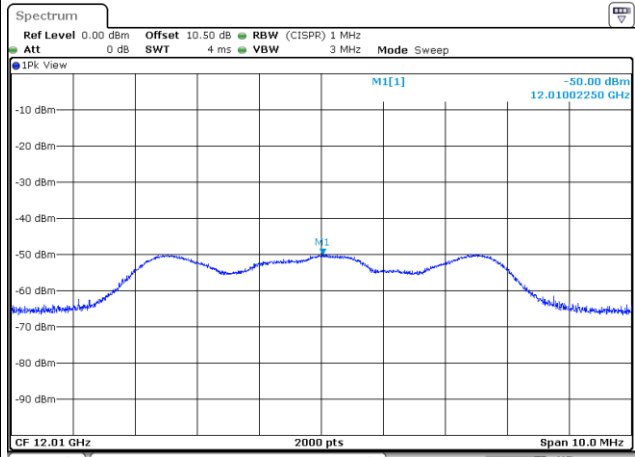
12010MHz - PK
