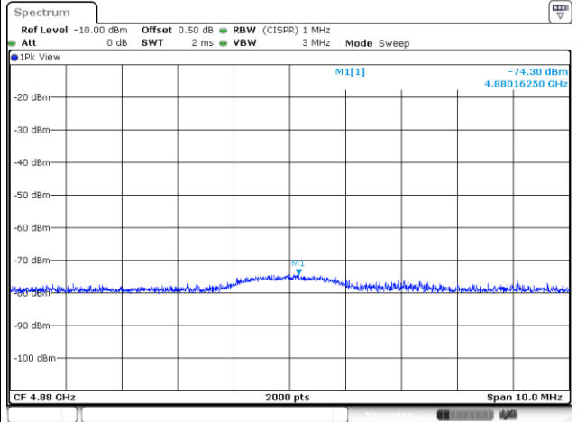
4880MHz - PK
