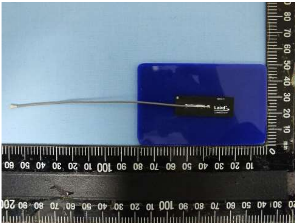
Ant.: EMF2471A3S-10MH4L
