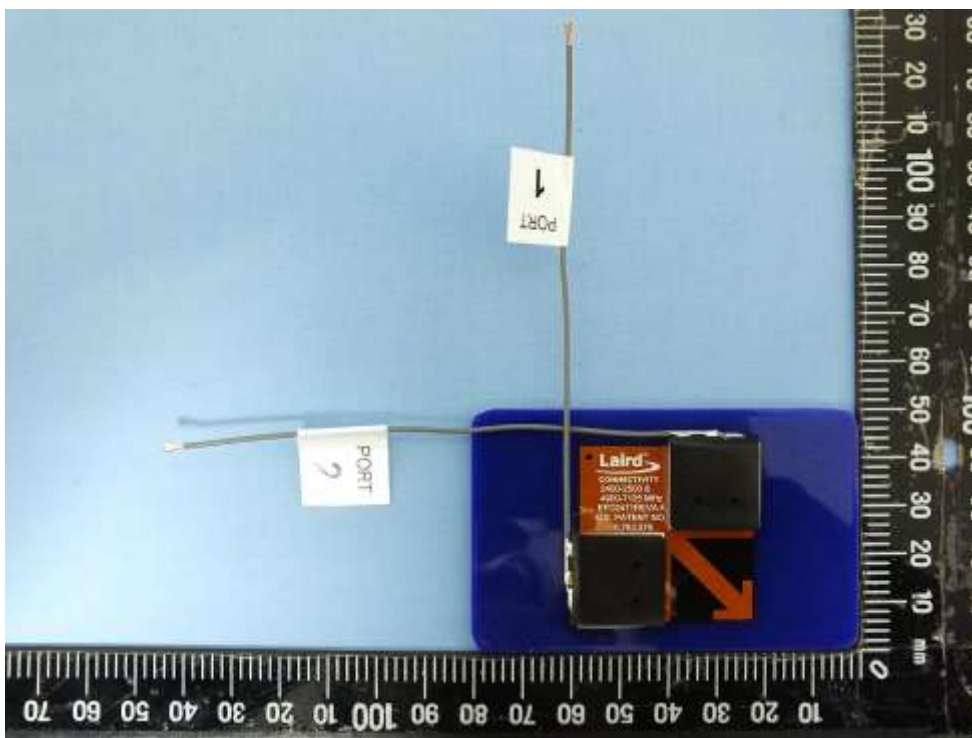
Ant.: EFD2471A3S-10MH4L
