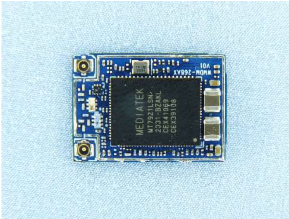
Ant.: EMF2471A3S-10MH4L
