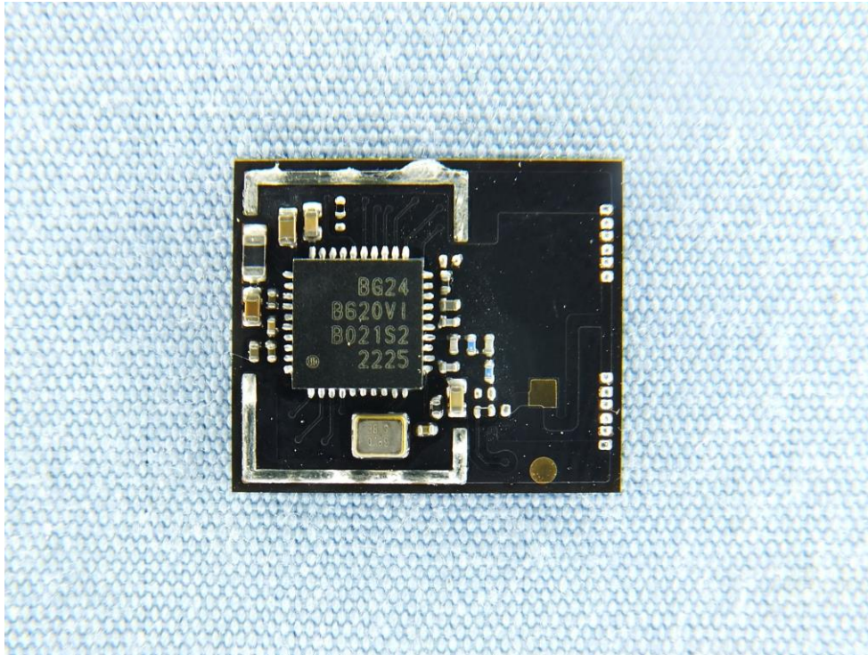
FlexPIFA antenna
