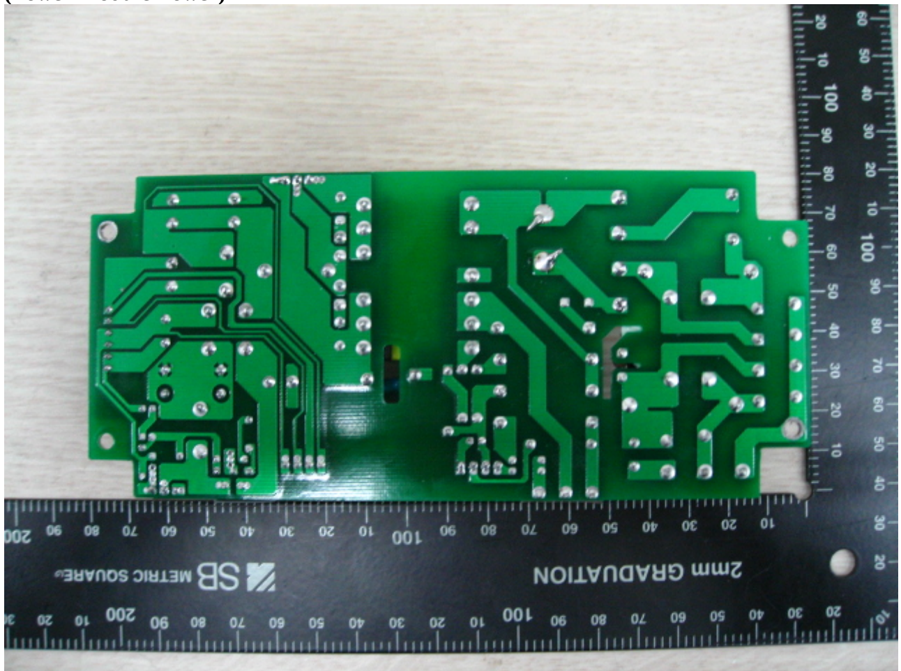
(Power Module Lower)
