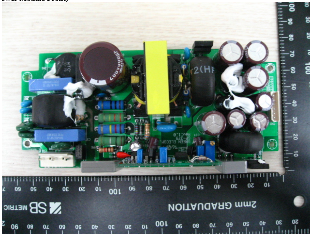
(Power Module Front)
