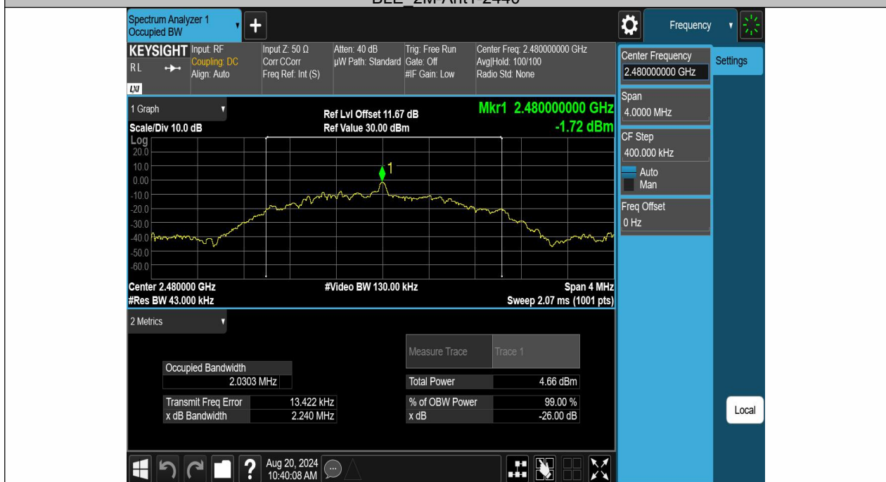
BLE_2M-Ant1-2480
