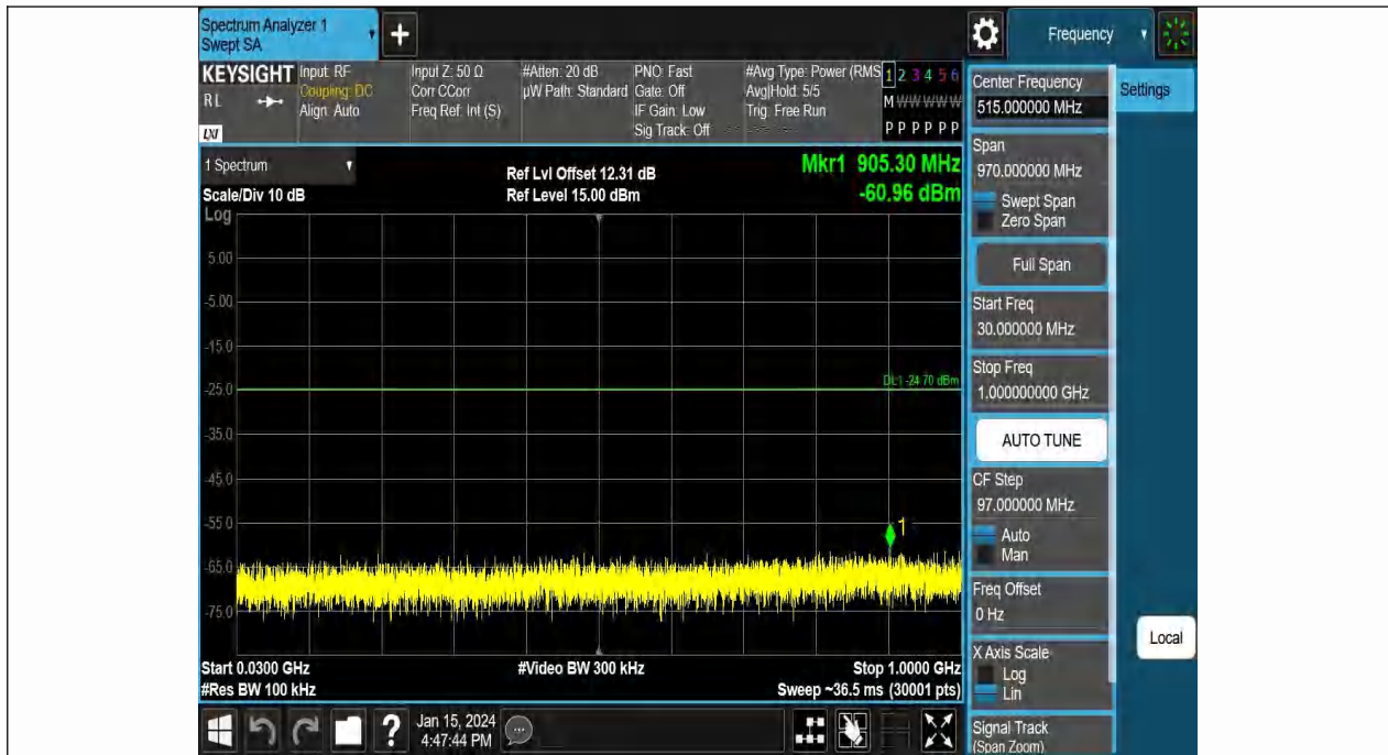
BLE_2M-Ant1-2402-30~1000-PASS
