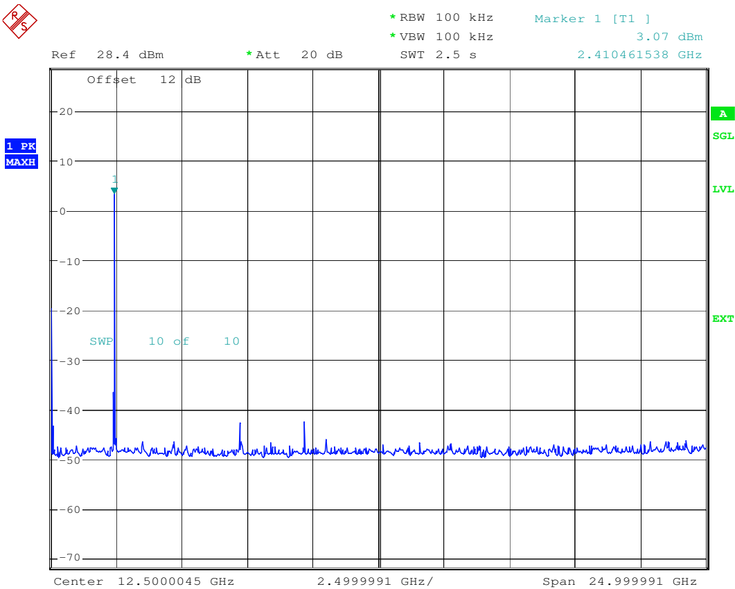
Plot 4: (OFDM)
