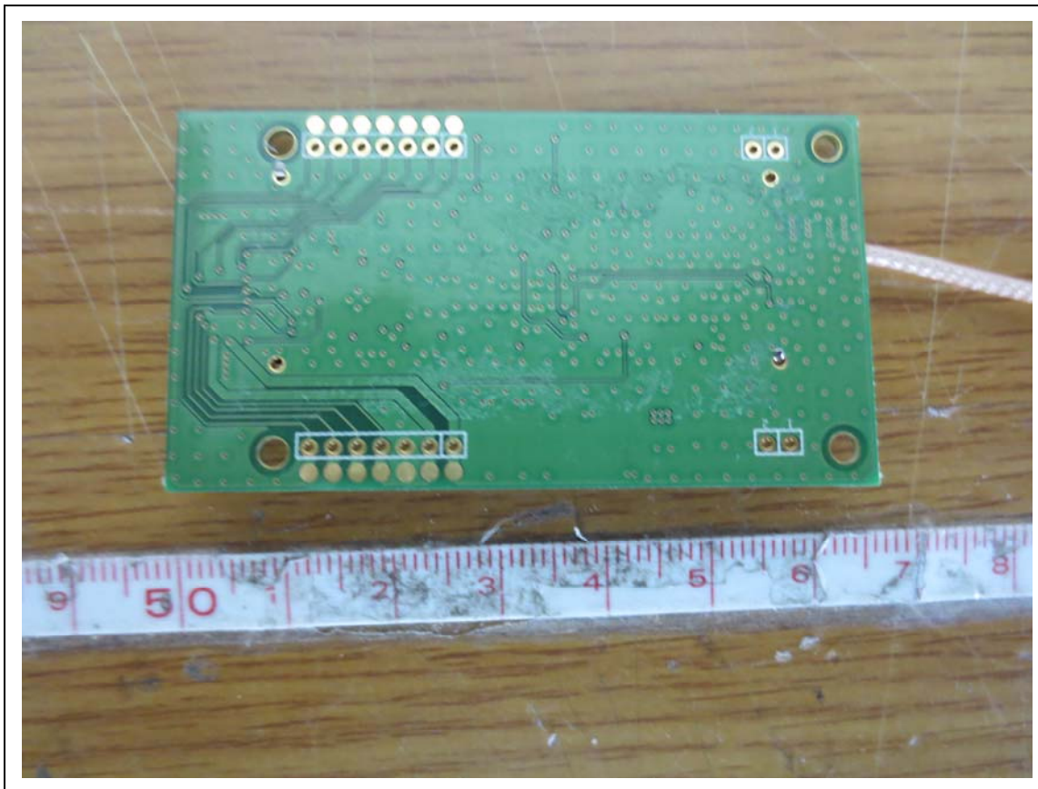
Module - Rear
