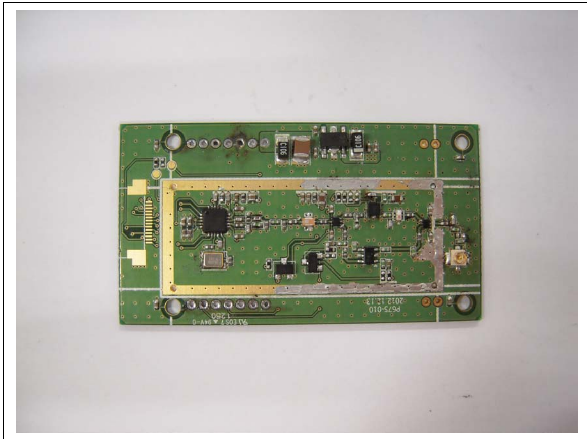
Module - Rear
