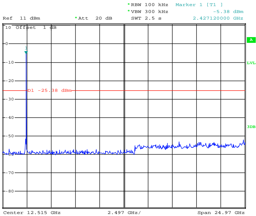
(Plot 4.6.2 A: Channel 1: 2412MHz @ 802.11g)
