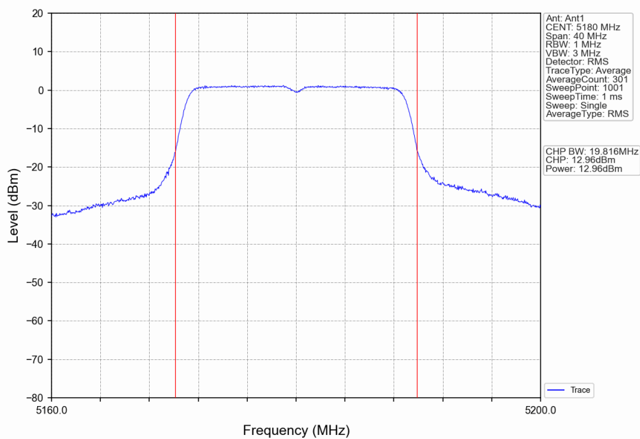
802.11n(HT20)_LCH_5180MHz_Ant1_NTN
