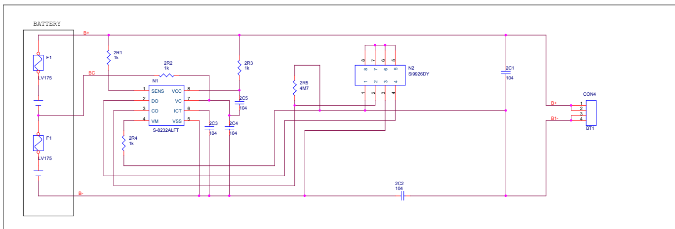
PD57001/PD57002/PD57003/PD58001/PD58002/PD59001/PD59002的保护板原理图 06年7, 8, 8.5寸PDVD保护板电路
