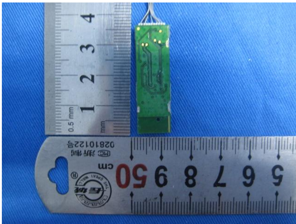
Bluetooth Module
