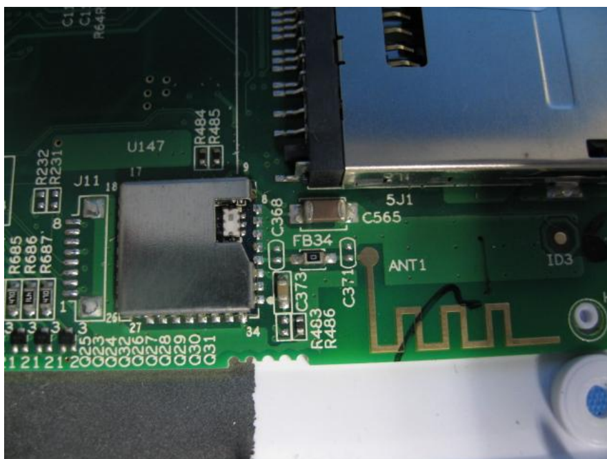
BT module
