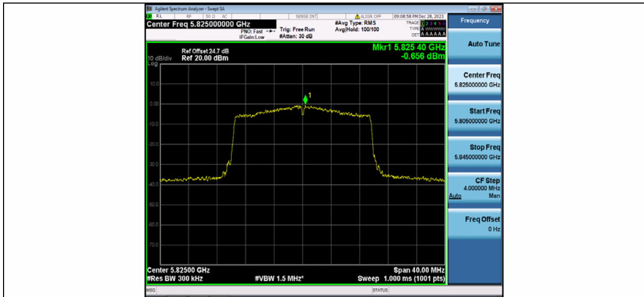
11AX20MIMO_Ant2_5825
