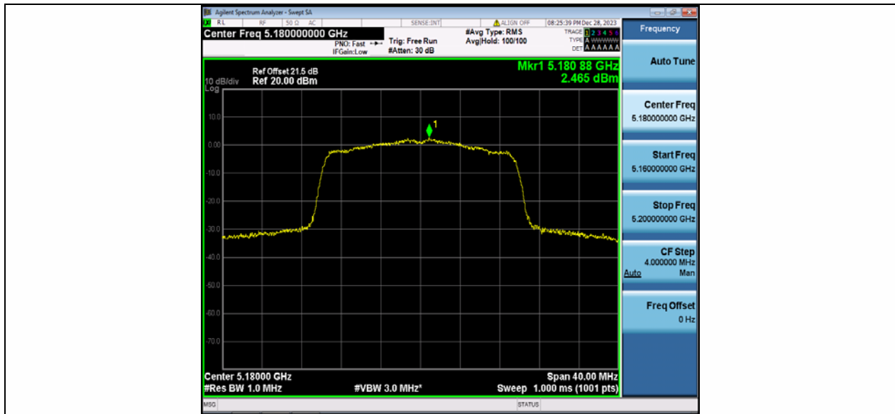
11AX20MIMO_Ant2_5180
