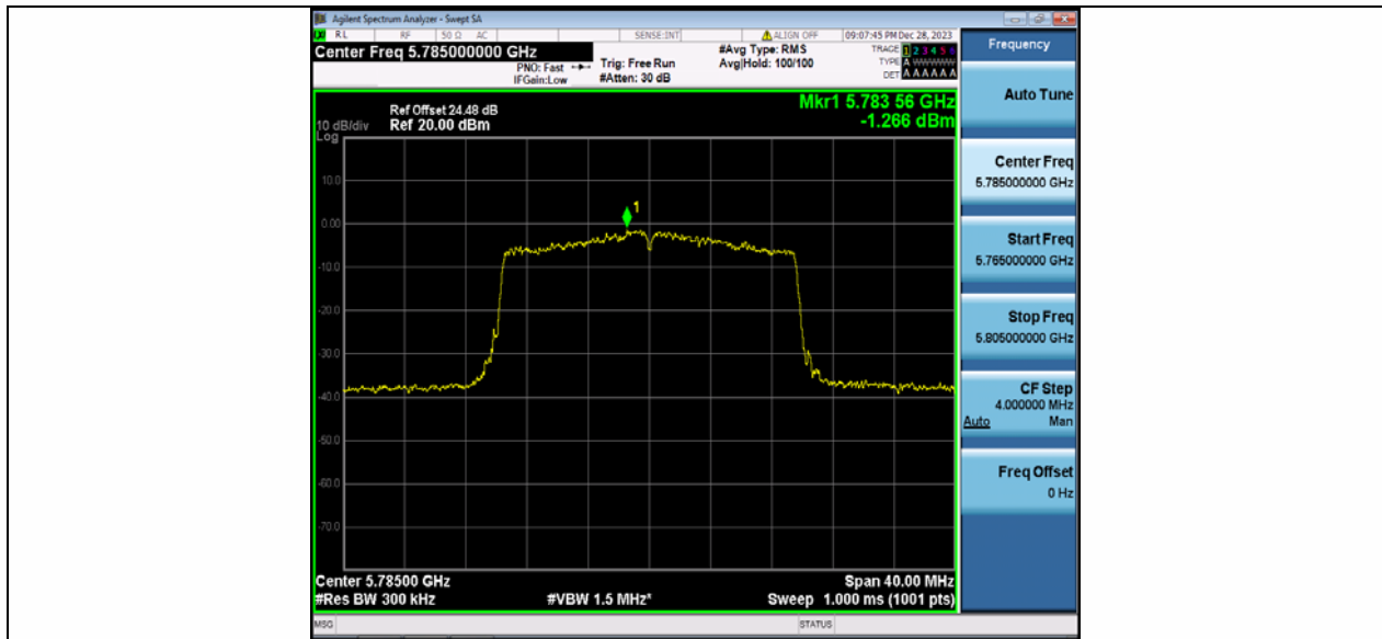
11AX20MIMO_Ant2_5785
