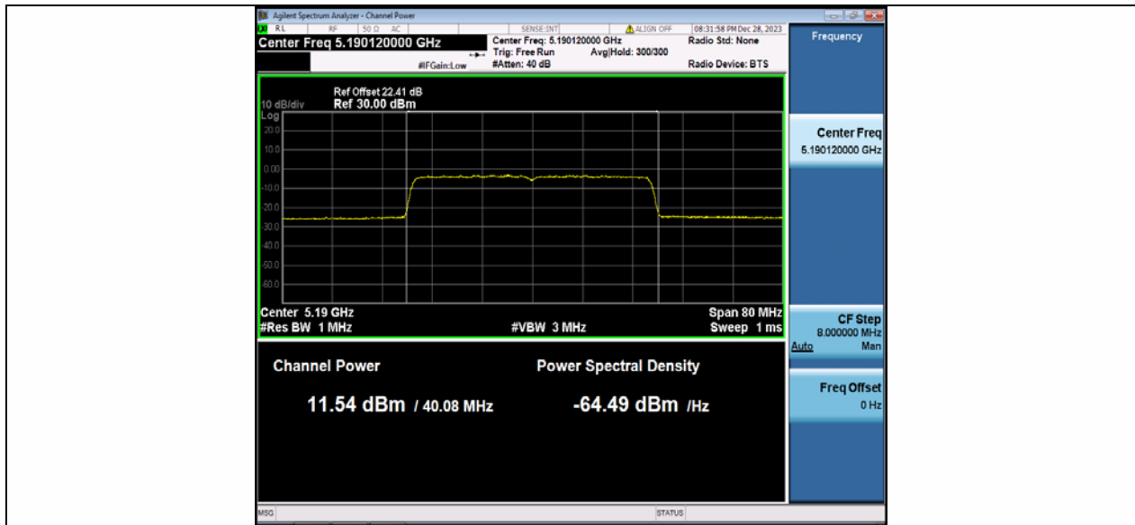
11AX40MIMO_Ant2_5190
