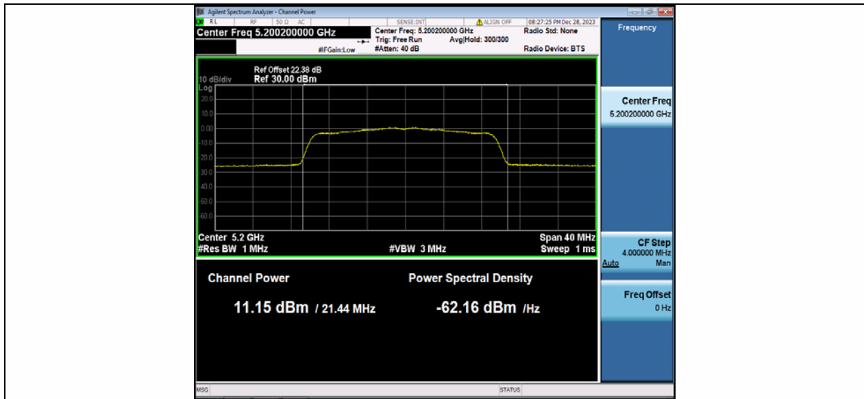
11AX20MIMO_Ant2_5200
