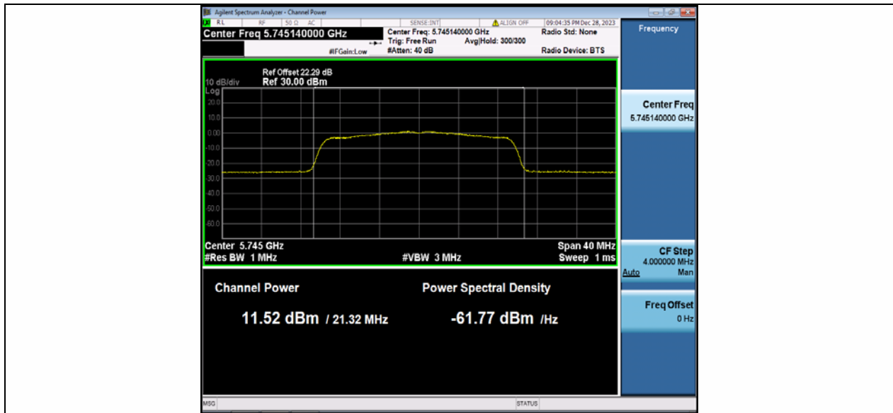
11AX20MIMO_Ant2_5745
