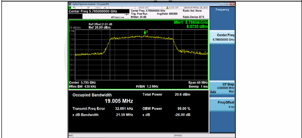
11AX20MIMO_Ant1_5785
