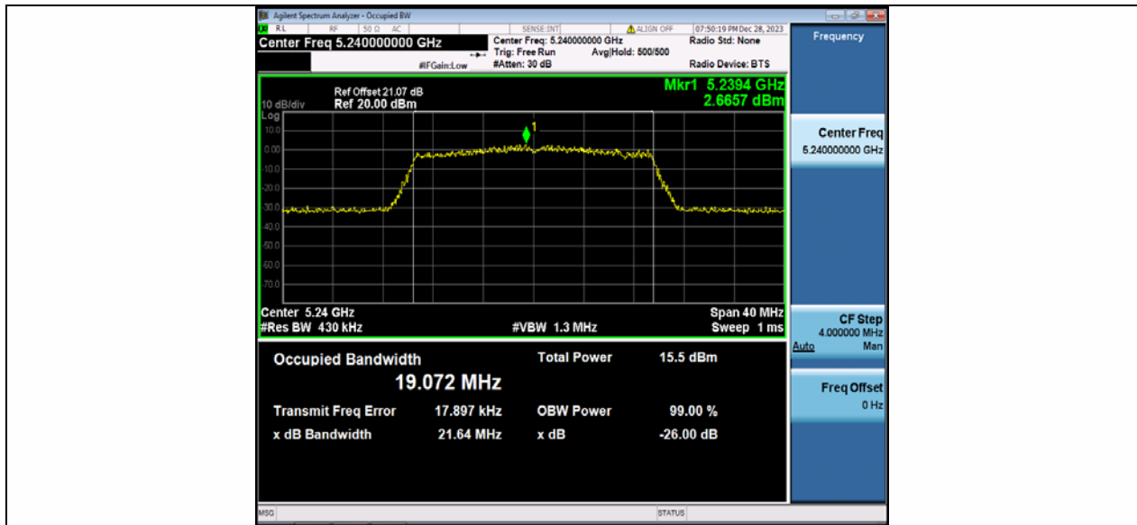
11AX20MIMO_Ant2_5240
