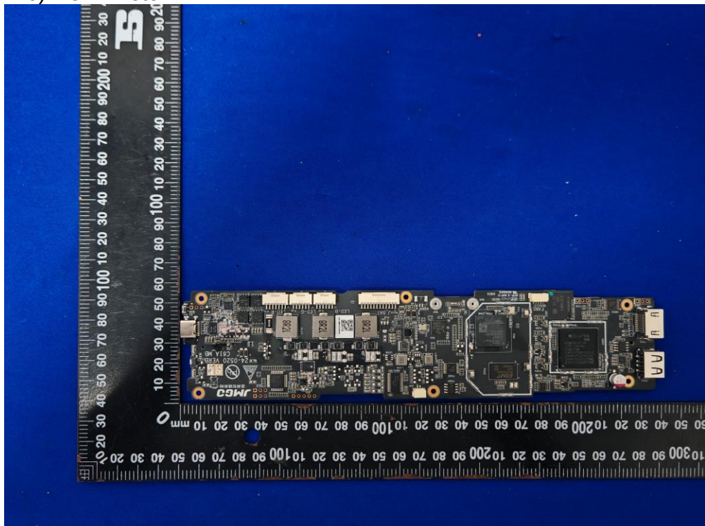
16) EUT Photo
