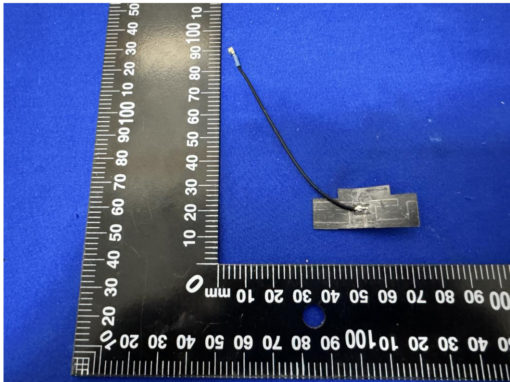
28) EUT Photo
