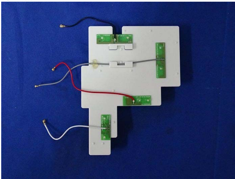
(30) EUT Photo
