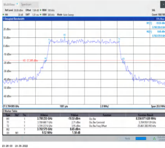
1-N78-3700-3800-30-10-L-9-CP-256QAM-Outer_Full -24@0-Ant1-8.557-9.520-≤10-PASS
