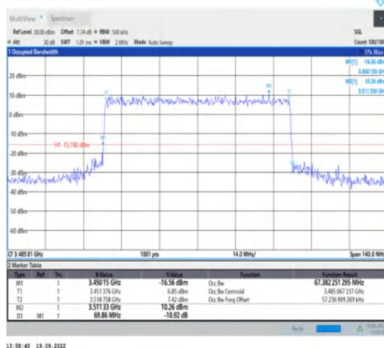
1-N78-3450-3550--30-70-L-6-CP-QPSK-Outer_Full-1 89@0-Ant1-67.382-69.860-≤70-PASS
