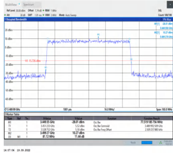
1-N78-3450-3550--30-80-L-9-CP-256QAM-Outer_Fu ll-217@0-Ant1-77.519-81.120-≤80-PASS
