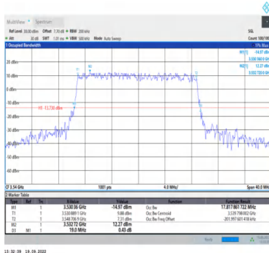
1-N78-3450-3550--30-20-H-4-DFT-64QAM-Outer_Fu II-50@0-Ant1-17.818-19.000-≤20-PASS
