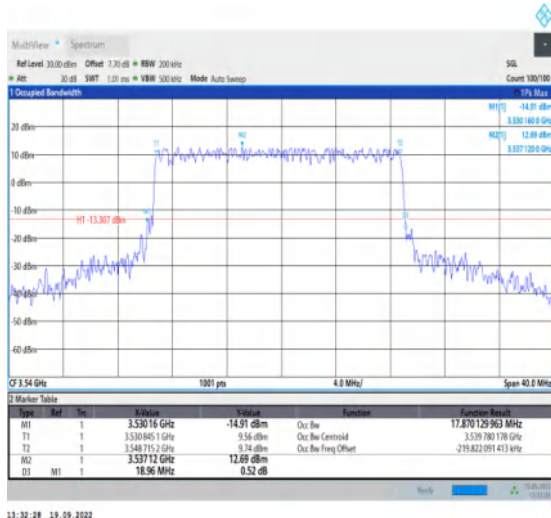
1-N78-3450-3550--30-20-H-3-DFT-16QAM-Outer_Fu II-50@0-Ant1-17.87-18.960-≤20-PASS
