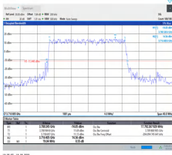
1-N77-3700-3980--30-20-L-2-DFT-PI2BPSK-Outer_F ull-50@0-Ant1-17.792-19.040-≤20-PASS
