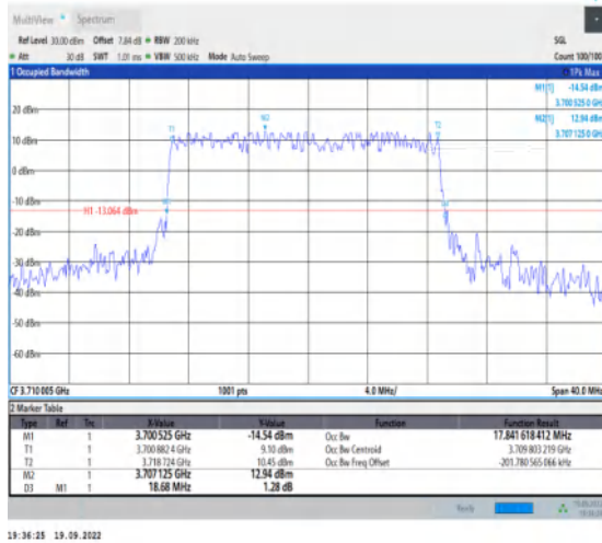
1-N77-3700-3980--30-20-L-3-DFT-16QAM-Outer_Fu I-50@0-Ant1-17.842-18.680-≤20-PASS
