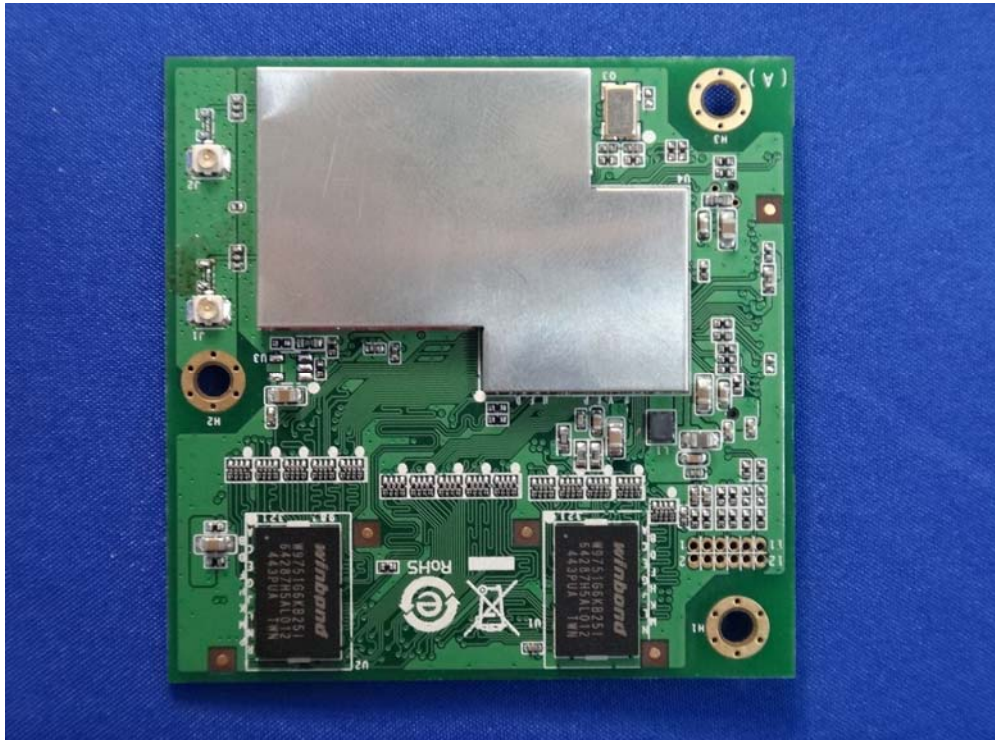
(17) EUT Photo
