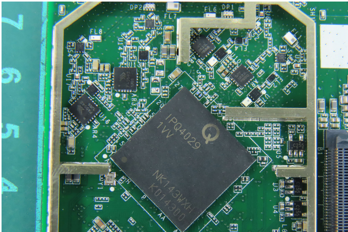
(50) EUT Photo
