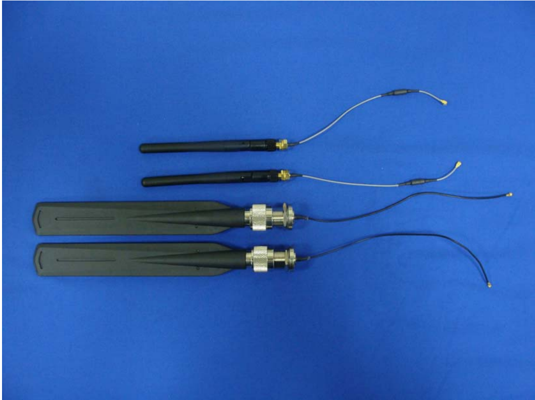
(5) EUT Photo
