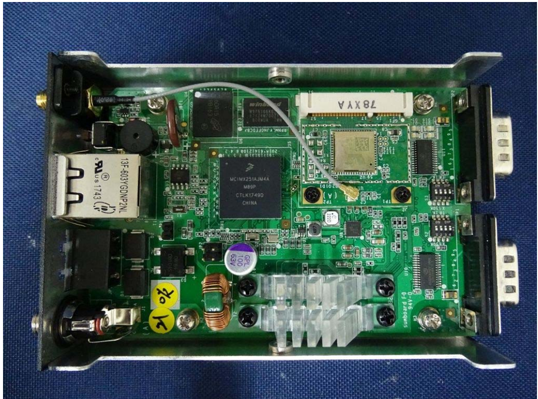
(15) EUT Photo
