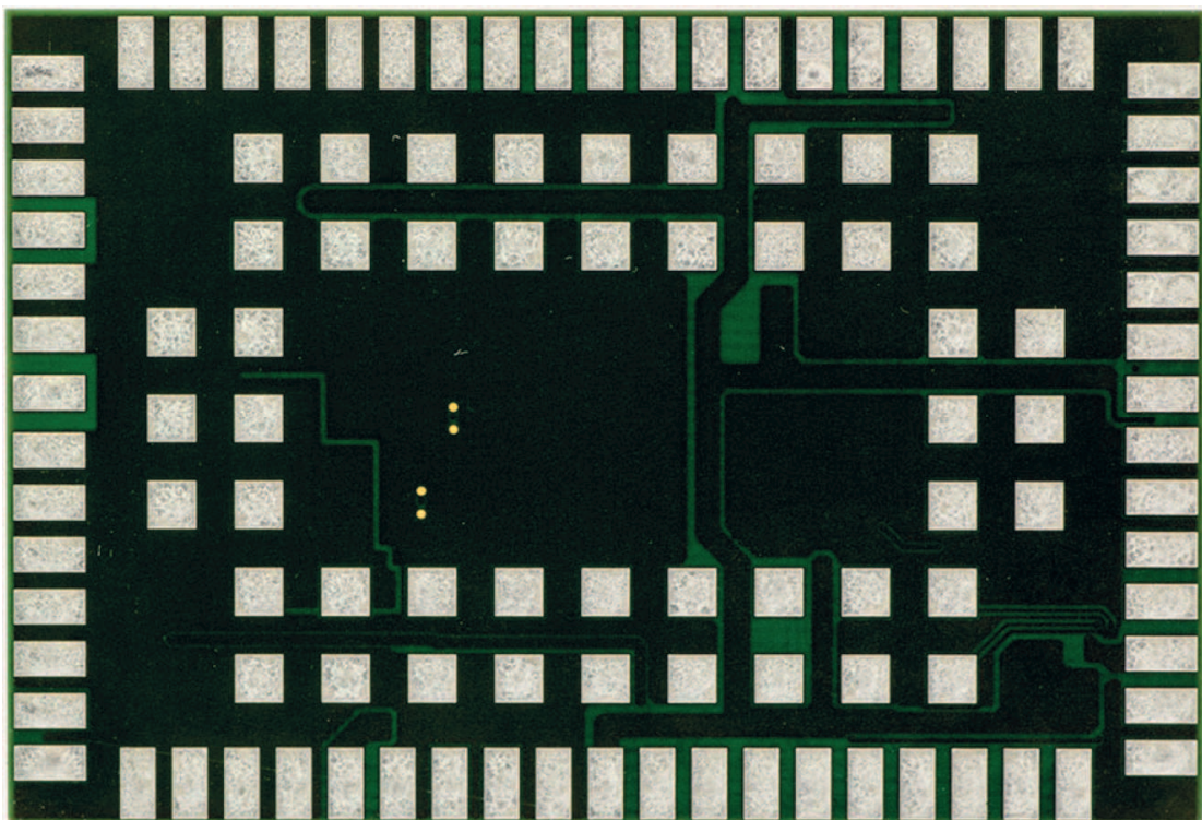
Bottom Side
