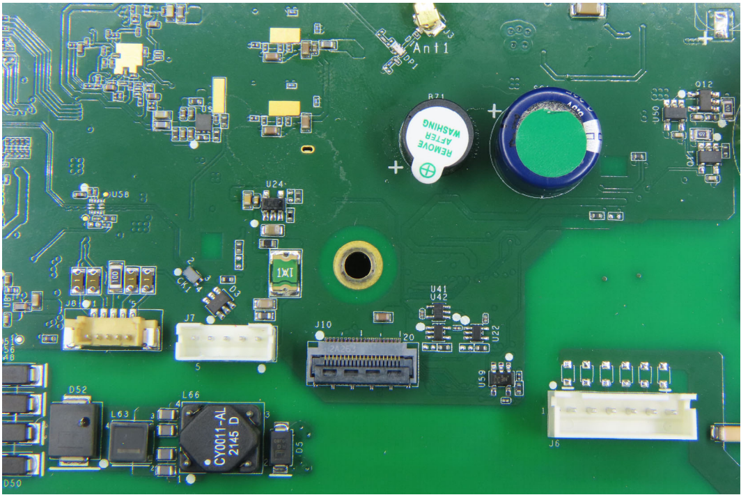
(44) EUT Photo
