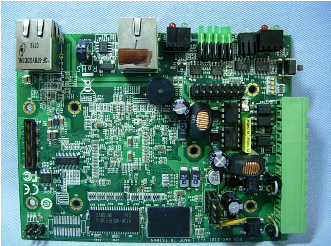
(18) EUT Photo
