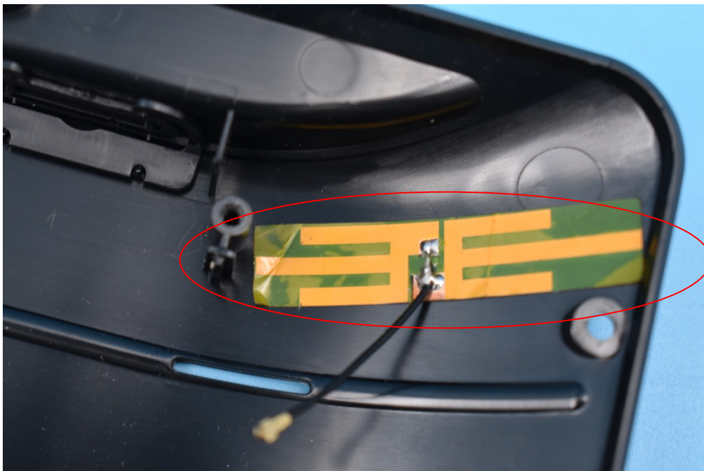
4. BT/WIFI antenna view
