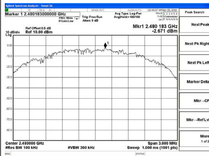
2479 – 2481 MHz
