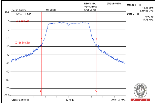
802.11n (40MHz)
