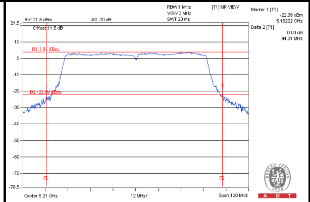
802.11ac (VHT80)
