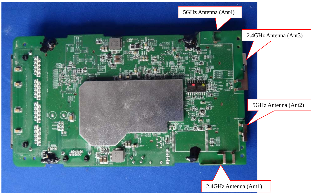
(19) EUT Photo
