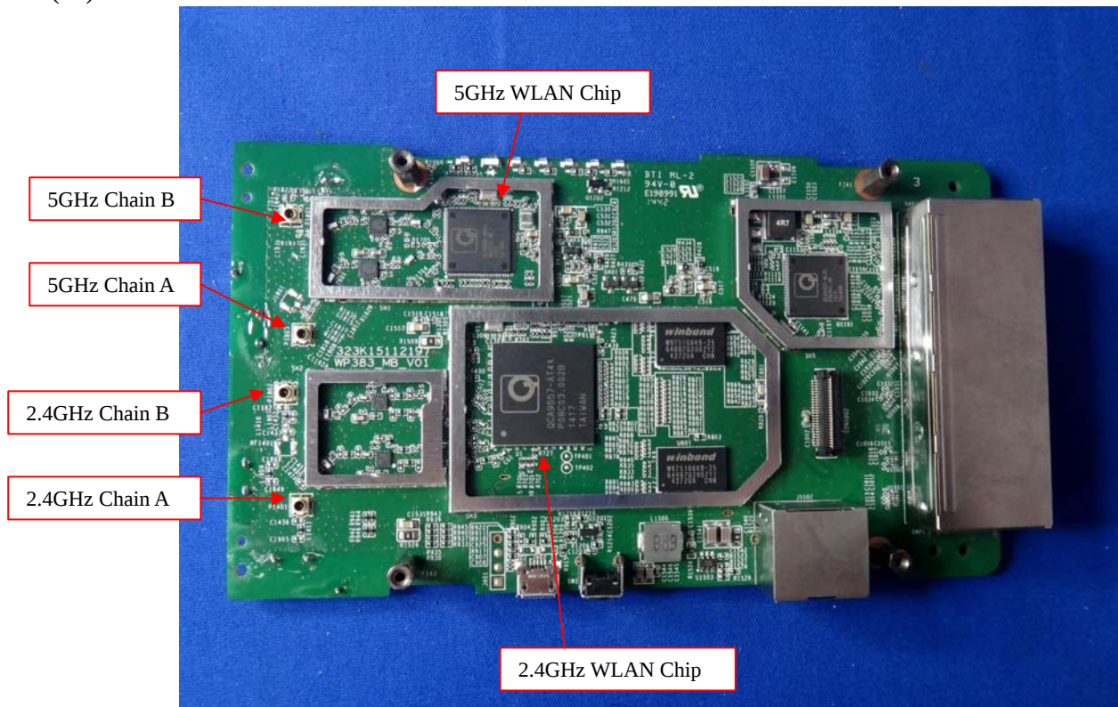
(15) EUT Photo
