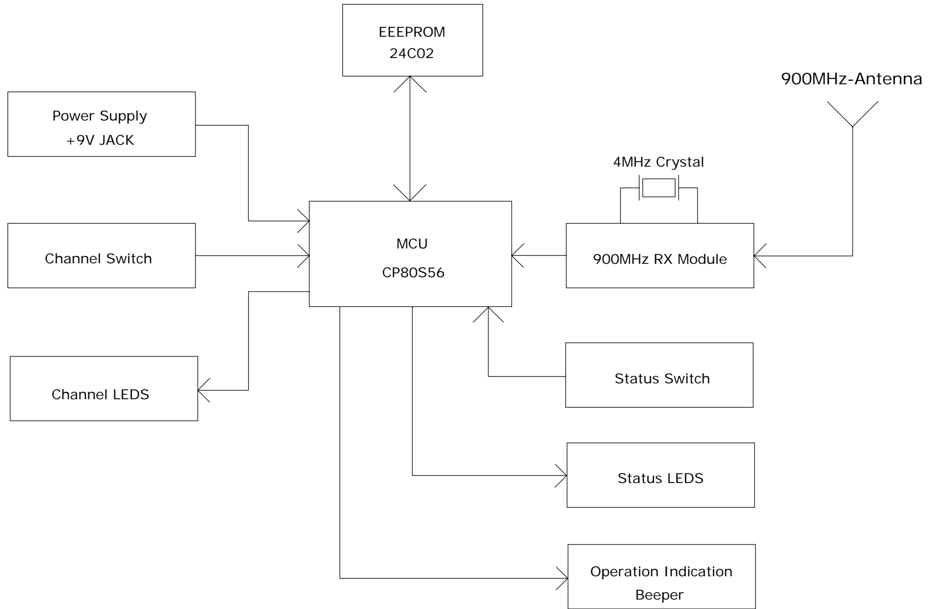
Figure1 RX160-900MHz Block Diagram
