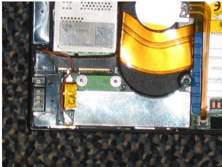
WLAN Module
